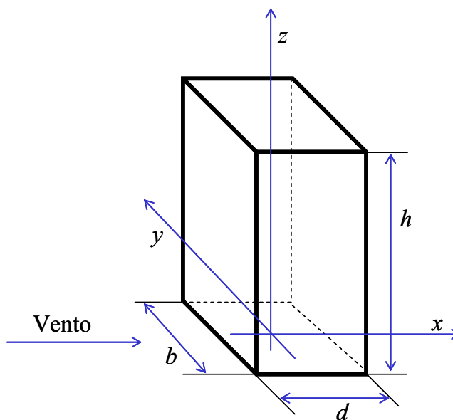
Figura 4.6.1 - Edificio C.A.A.R.C.
