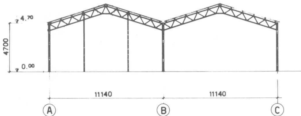
Figura 4.8.2 – Sezione W-W della tettoia.
