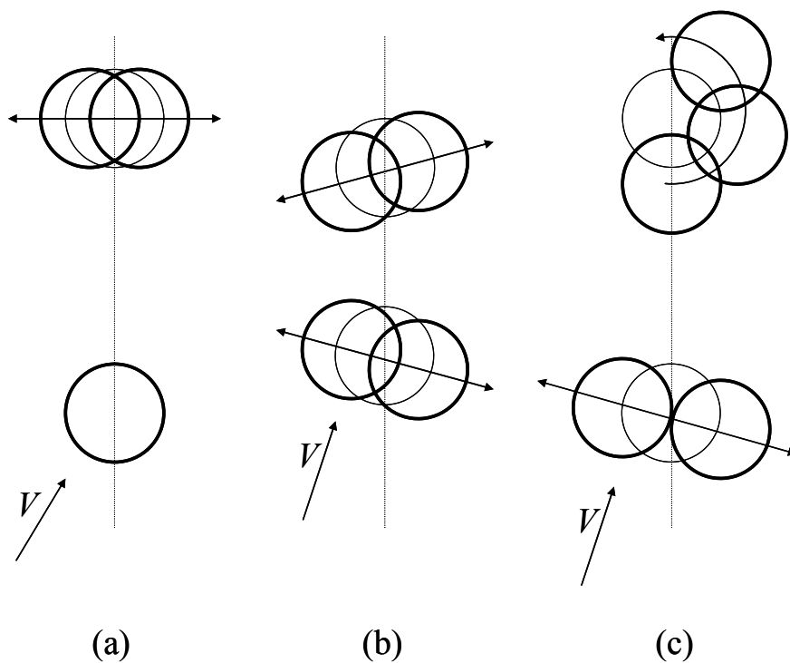
Figura 2.36 - Interferenza aeroelastica associata al galoppo indotto da una scia vorticosi.
